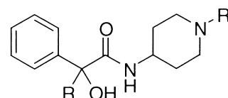
4 4-acetamidopiperidines
