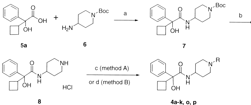
Scheme 1. Conditions: (a) WSC–HCl, HOBT, \text{CHCl}_3 ; (b) HCl–MeOH; (c) mesylate or halide, \text{K}_2\text{CO}_3 , \text{CH}_3\text{CN} ; (d) aldehyde, \text{NaB}(\text{OAc})_3\text{H} , THF.
